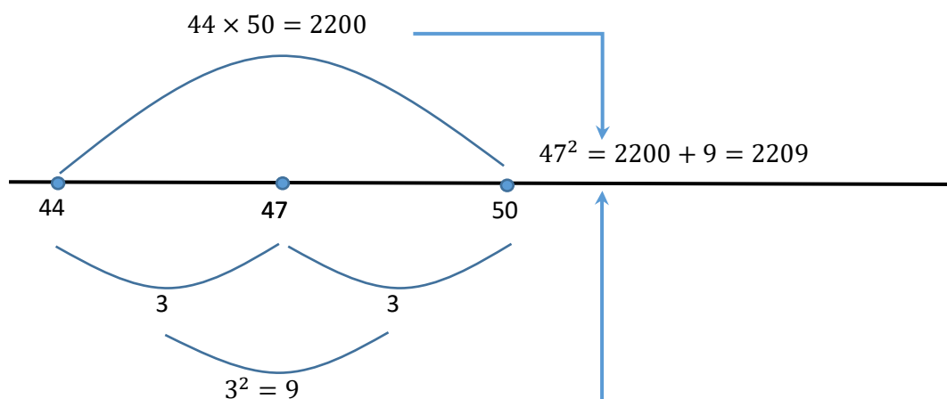
Gambar 2. Diagram Pengkuadratan bilangan 47^2
